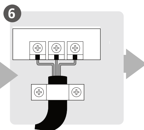
6 Povežite elektroinstalacije (Ne važi za neke lokacije u Severnoj Americi)
