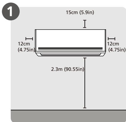
1 Izaberite lokaciju montaže
